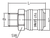
Male Thread Coupling Kupplung mit Aussengewinde
