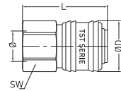
Female Thread Coupling Kupplung mit Innengewinde
