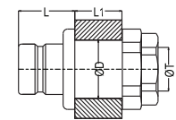
Built-in Plug Verschlussnippel mit Schottverschraubung
