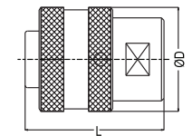
Female Threaded shut-off Plug Verschlussnippel mit Innengewinde
