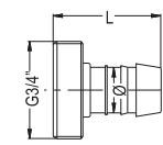
Male Thread Adapter With Hose Tail Aussengewinde Adapter mit Schlauchtülle
