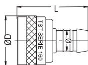
Coupling With Hose Tail Kupplung mit Schlauchtülle
